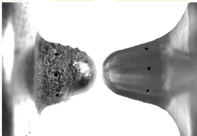
Injector diesel înainte și după curățare
